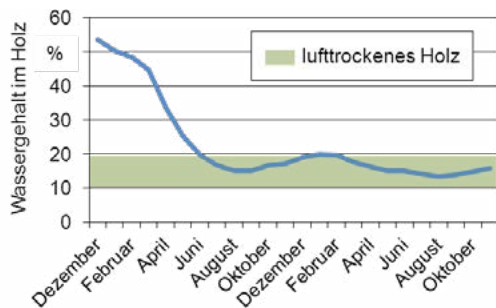
Beispiel für den Trocknungsverlauf von Scheitholz (gestapeltes, gespaltenes Meterholz, abgedeckt im Freien)
