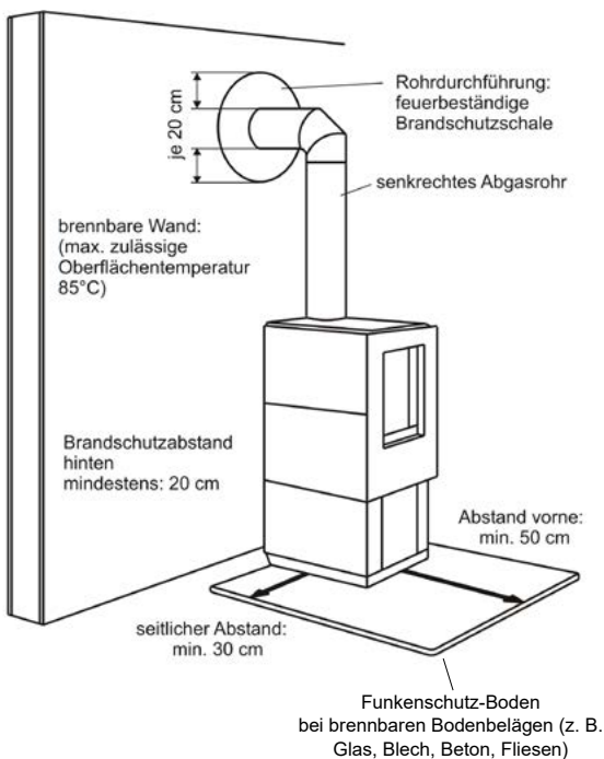
Sicherheitsabstände bei der Aufstellung von Kaminöfen im Wohnraum mit brennbaren Wänden und brennbaren Fußböden.
