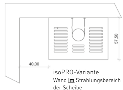
isoPRO-Variante Wand nicht im Strahlungsbereich der Scheibe
