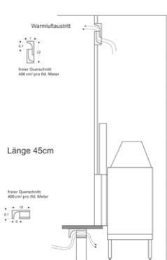
Warmluftleiste
