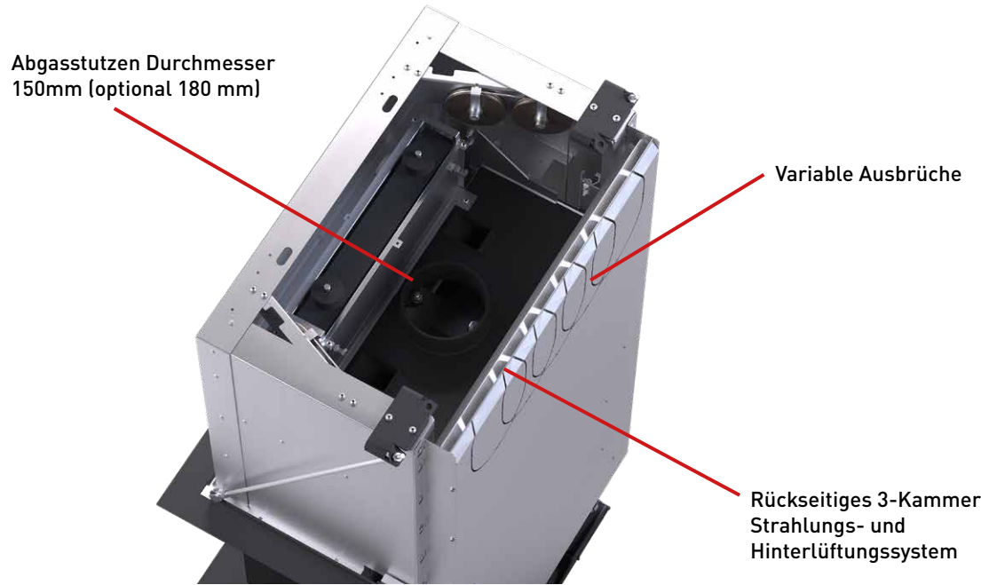
Abbildungen zeigen CB P200h - 8-seitiger massiver Blendrahmen
